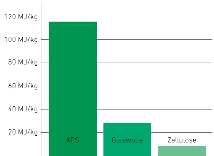
Primärenergieaufwand bei der Herstellung von Dämmstoffen im Vergleich. Quelle: TU Graz
